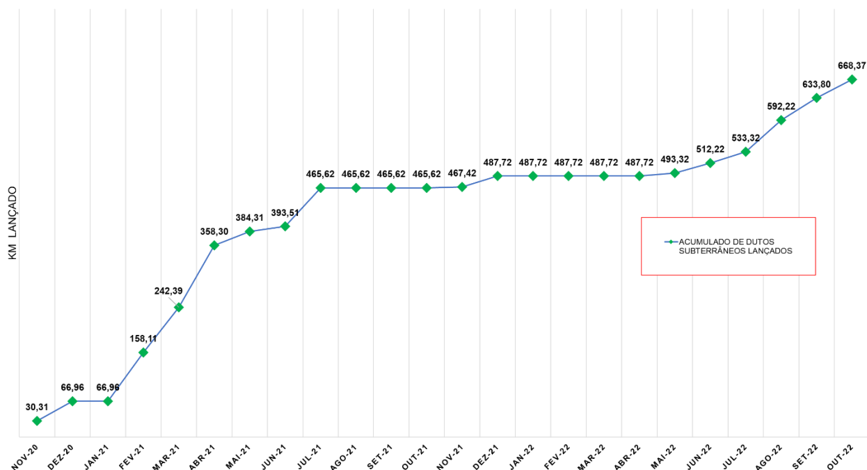
Figura 42 – Infraestrutura executada no backbone subterrâneo (Km)
