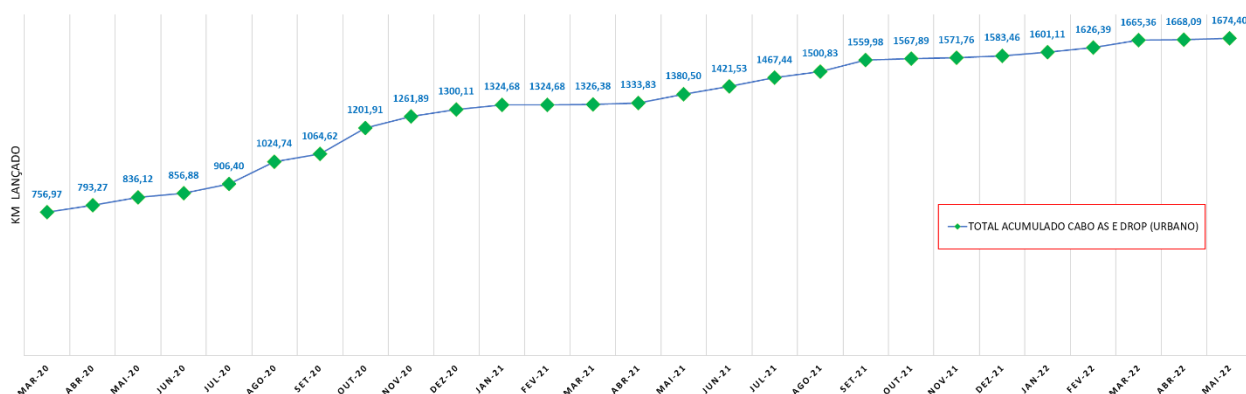
Figura 158 - Gráfico apresentando o acumulado de cabos da rede GPON concluídos até o mês de maio de 2022
