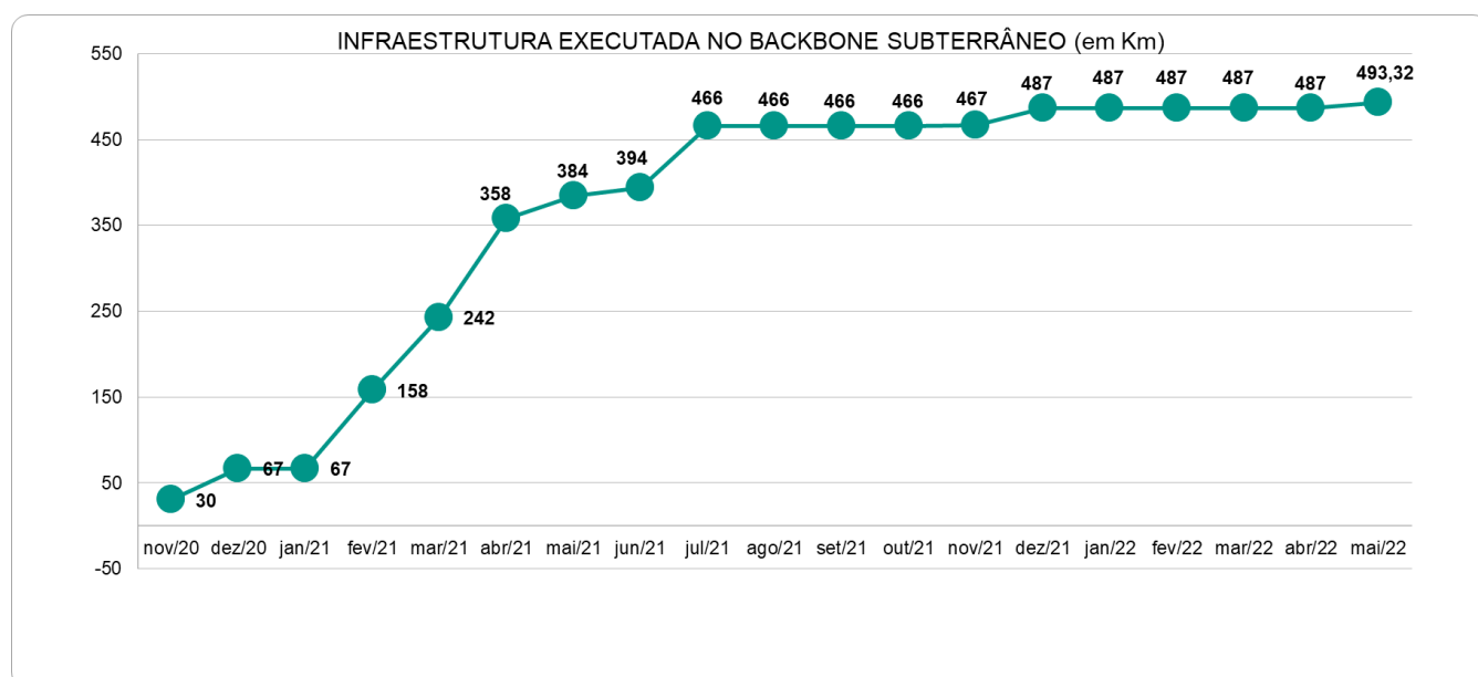
Figura 163 – Infraestrutura executada no backbone subterrâneo (Km)
