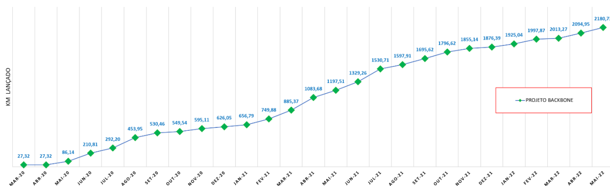
Figura 160 - Gráfico apresentando o acumulado de cabos de cabos do Backbone concluídos até o mês de maio de 2022
