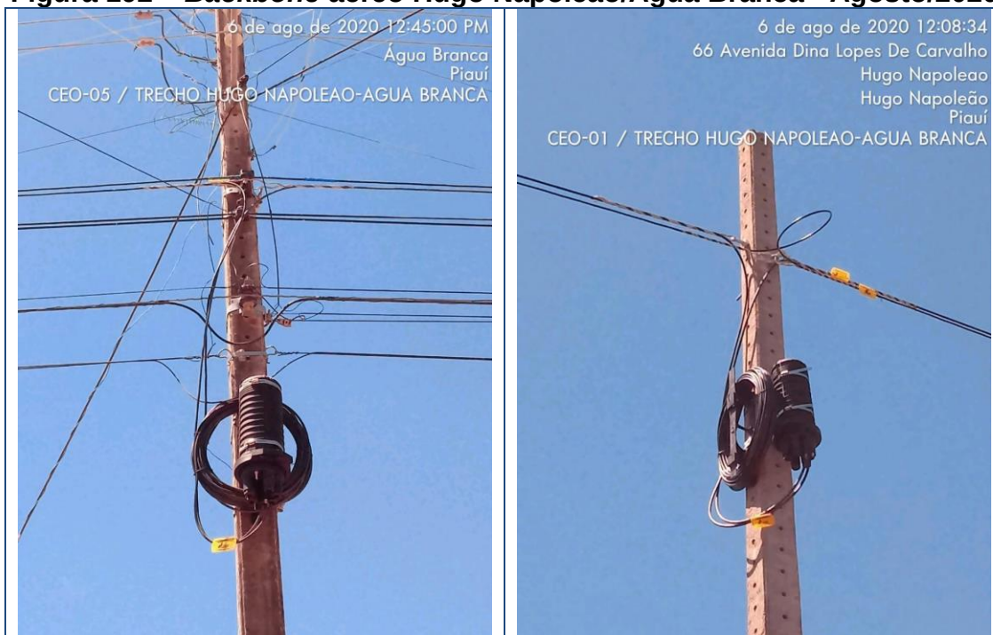
Figura 192 – Backbone aéreo Hugo Napoleão/Água Branca - Agosto/2020
