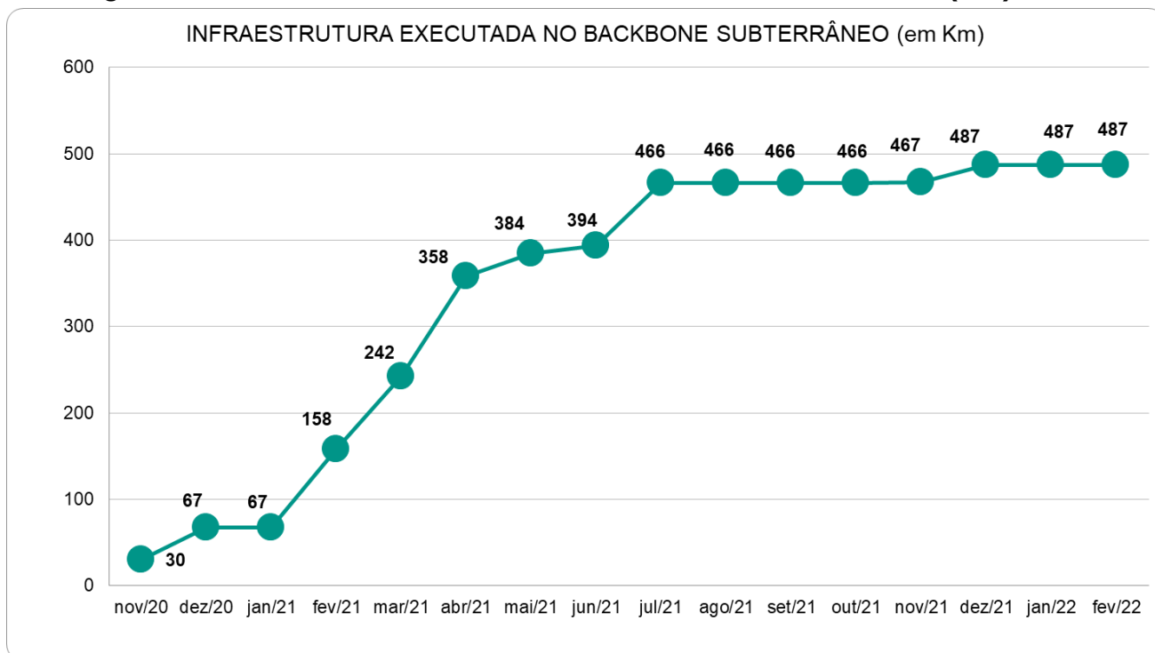
Figura 174 – Infraestrutura executada no backbone subterrâneo (Km)
