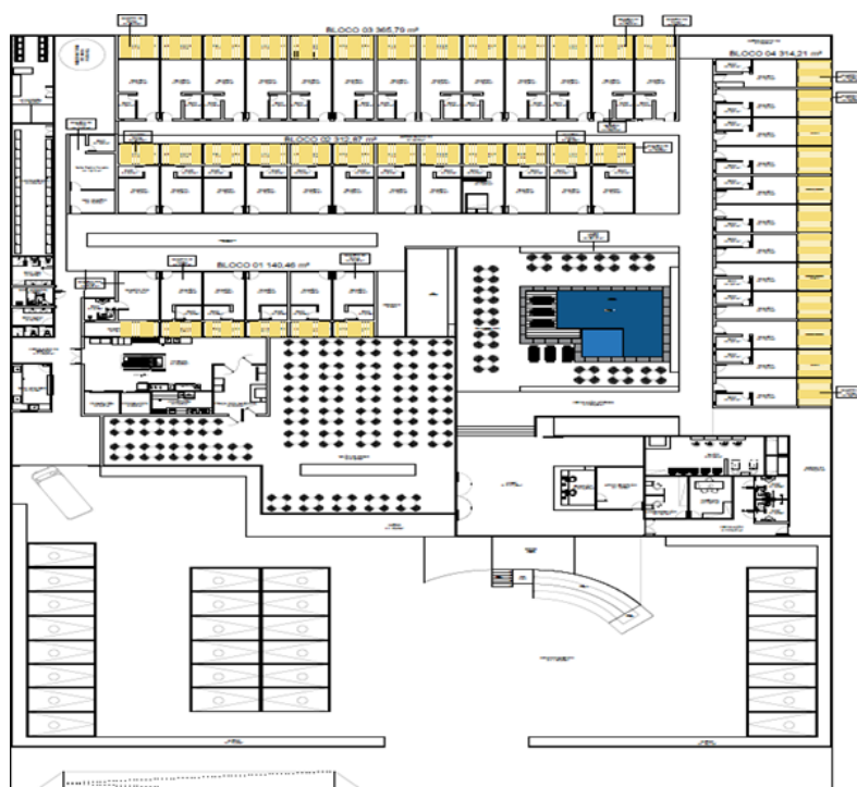
Figura 02 - Planta Baixa do Hotel
