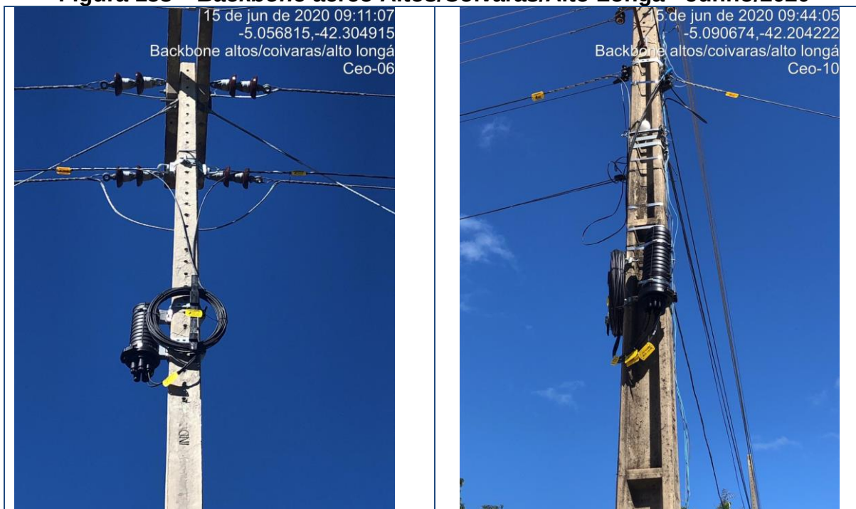
Figura 158 – Backbone aéreo Altos/Coivaras/Alto Longá - Junho/2020
