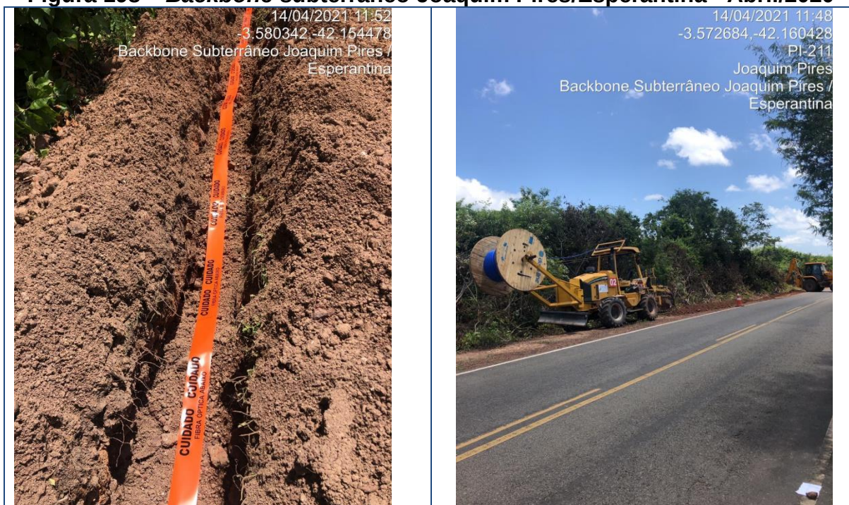
Figura 198 – Backbone subterrâneo Joaquim Pires/Esperantina - Abril/2020
