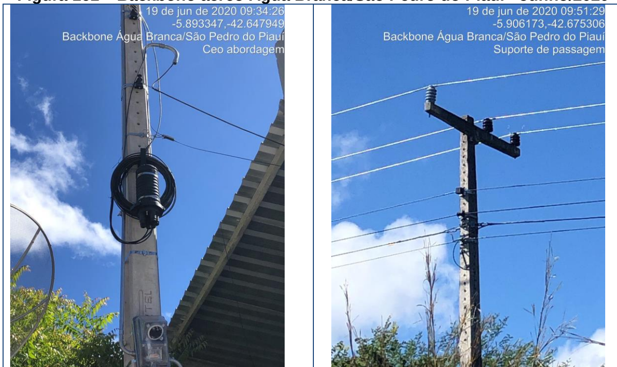
Figura 161 – Backbone aéreo Água Branca/São Pedro do Piauí - Junho/2020
