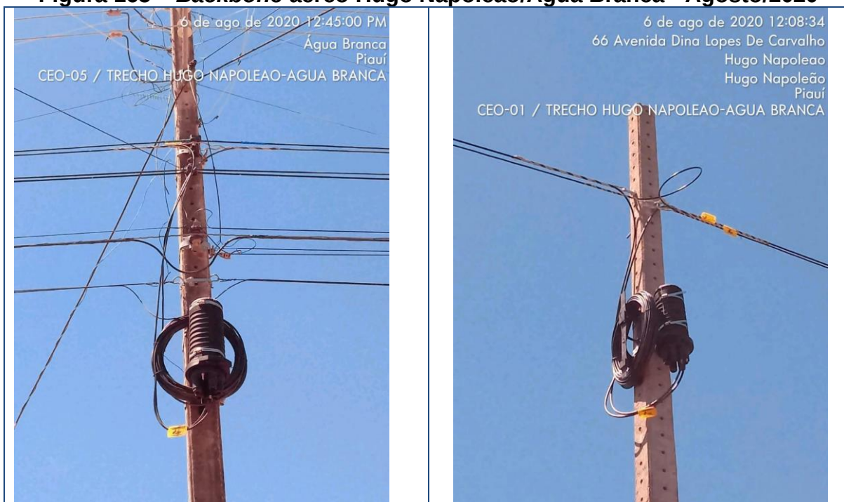
Figura 165 – Backbone aéreo Hugo Napoleão/Água Branca - Agosto/2020
