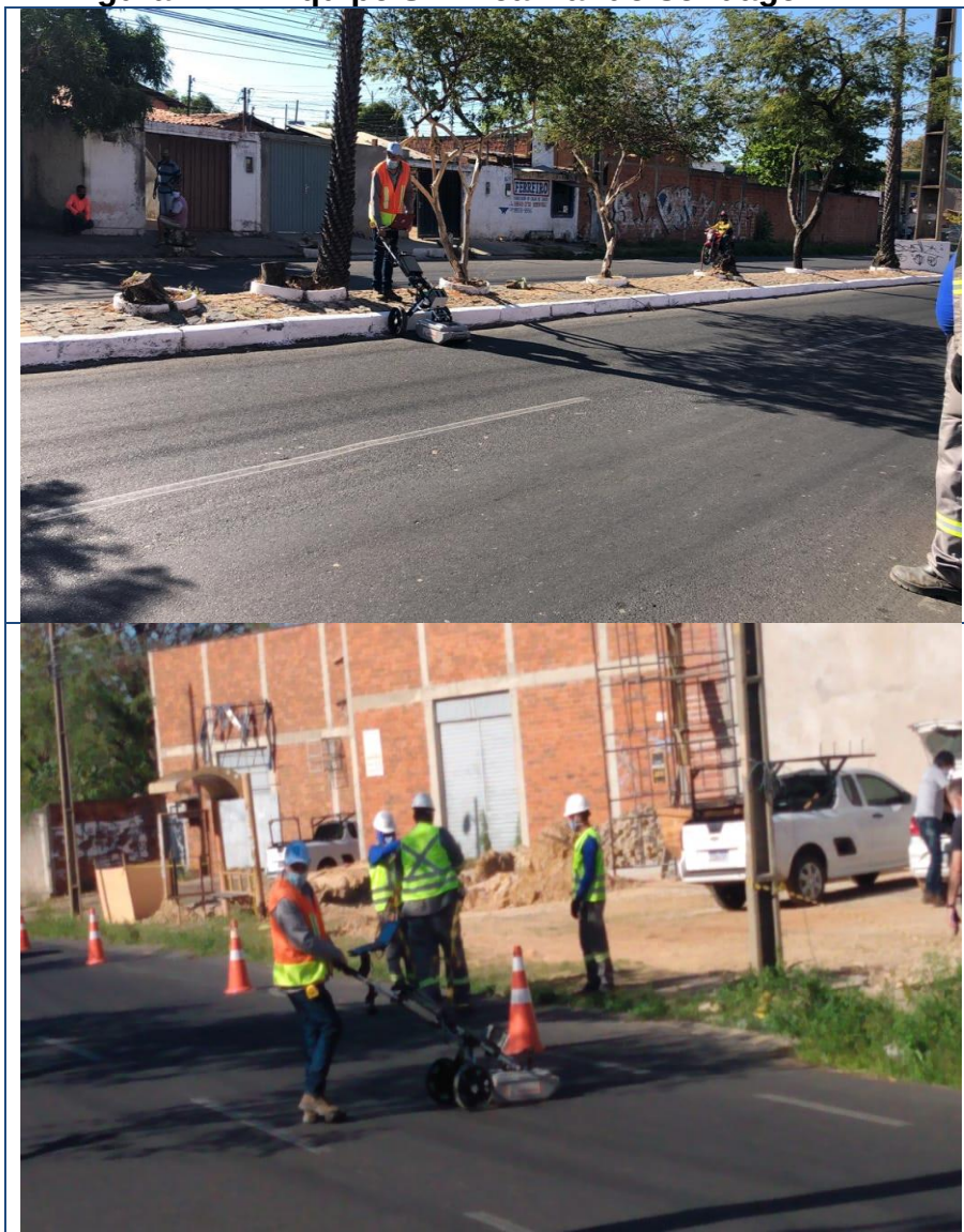
Figura 177 – Equipe SPE realizando sondagem MND
