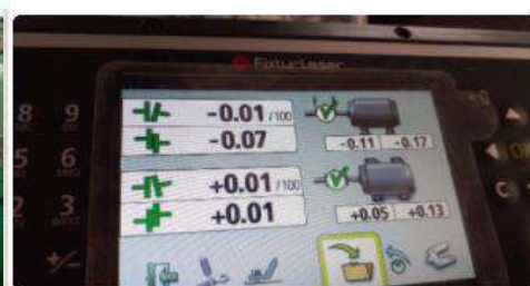
CMB 03 da ETA I alinhado
