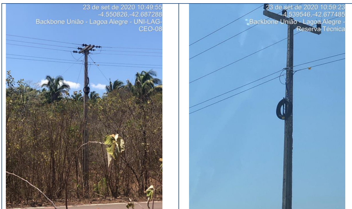
Figura 178 – Backbone aéreo União/Lagoa Alegre
