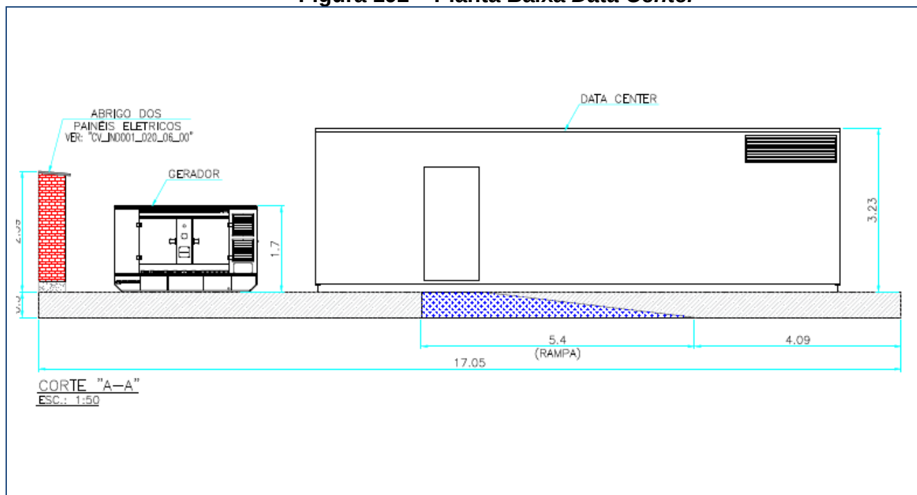
Figura 192 – Planta Baixa Data Center
