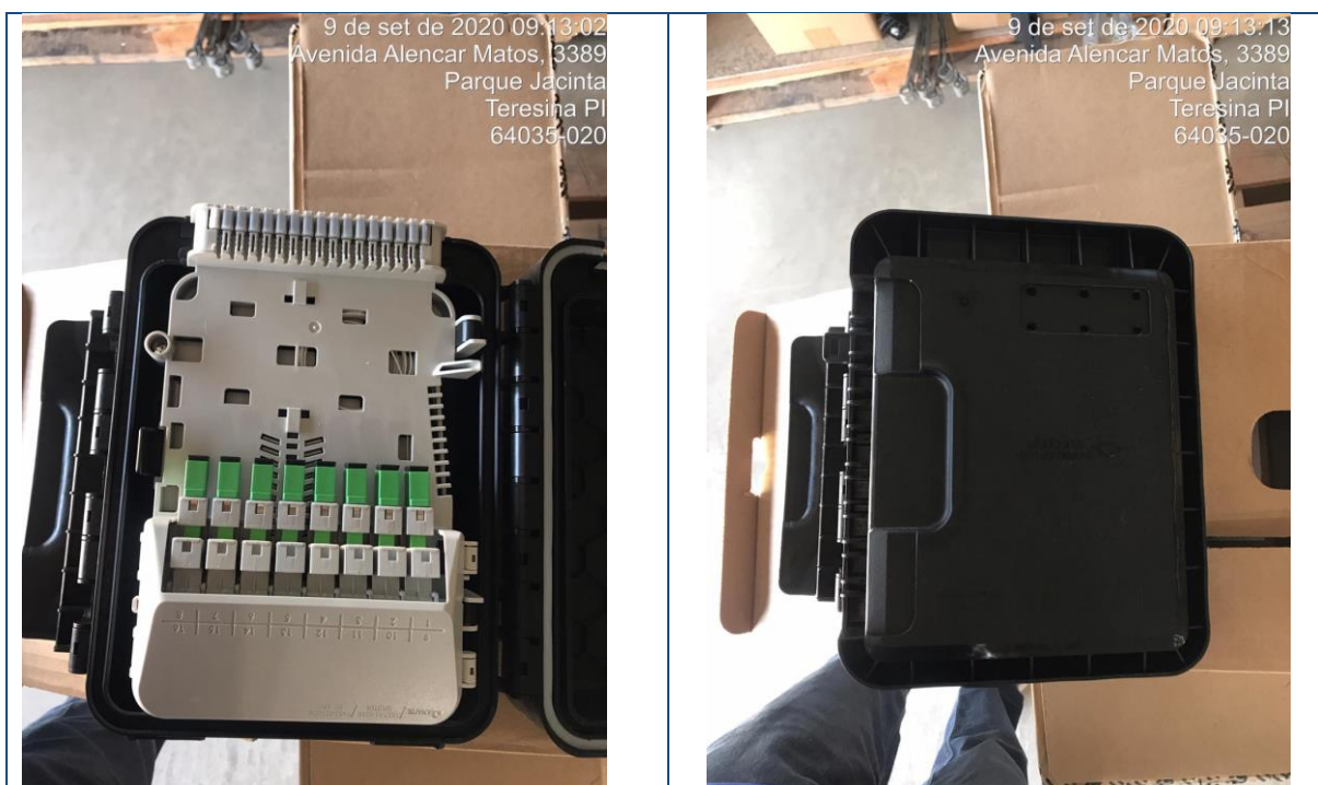
Figura 165 – Materiais e Equipamentos para implantação do Backbone
