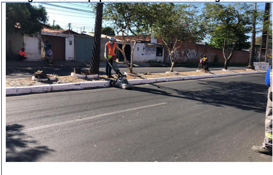
Figura 160 – Equipe SPE realizando sondagem MND
