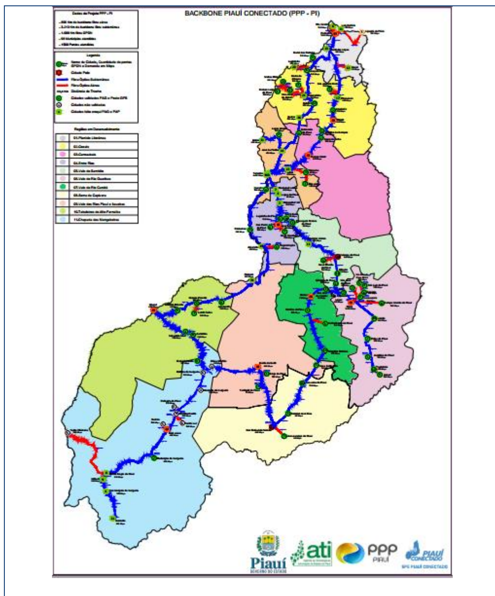
Figura 156 – Mapa de implantação do Backbone Piauí Conectado
