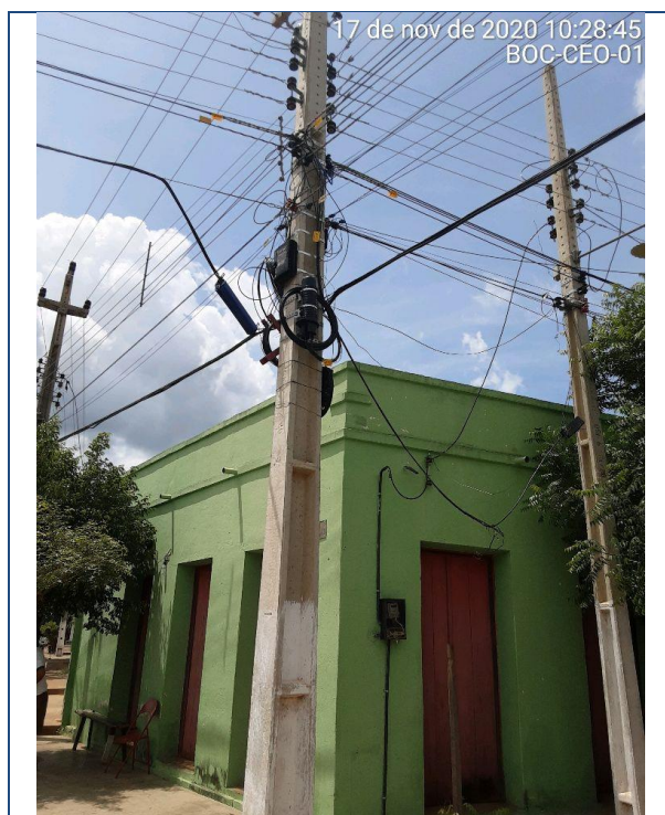
Figura 50 – BOC-CEO-01 – Reserva técnica aplicada não corretamente– Bocaina
