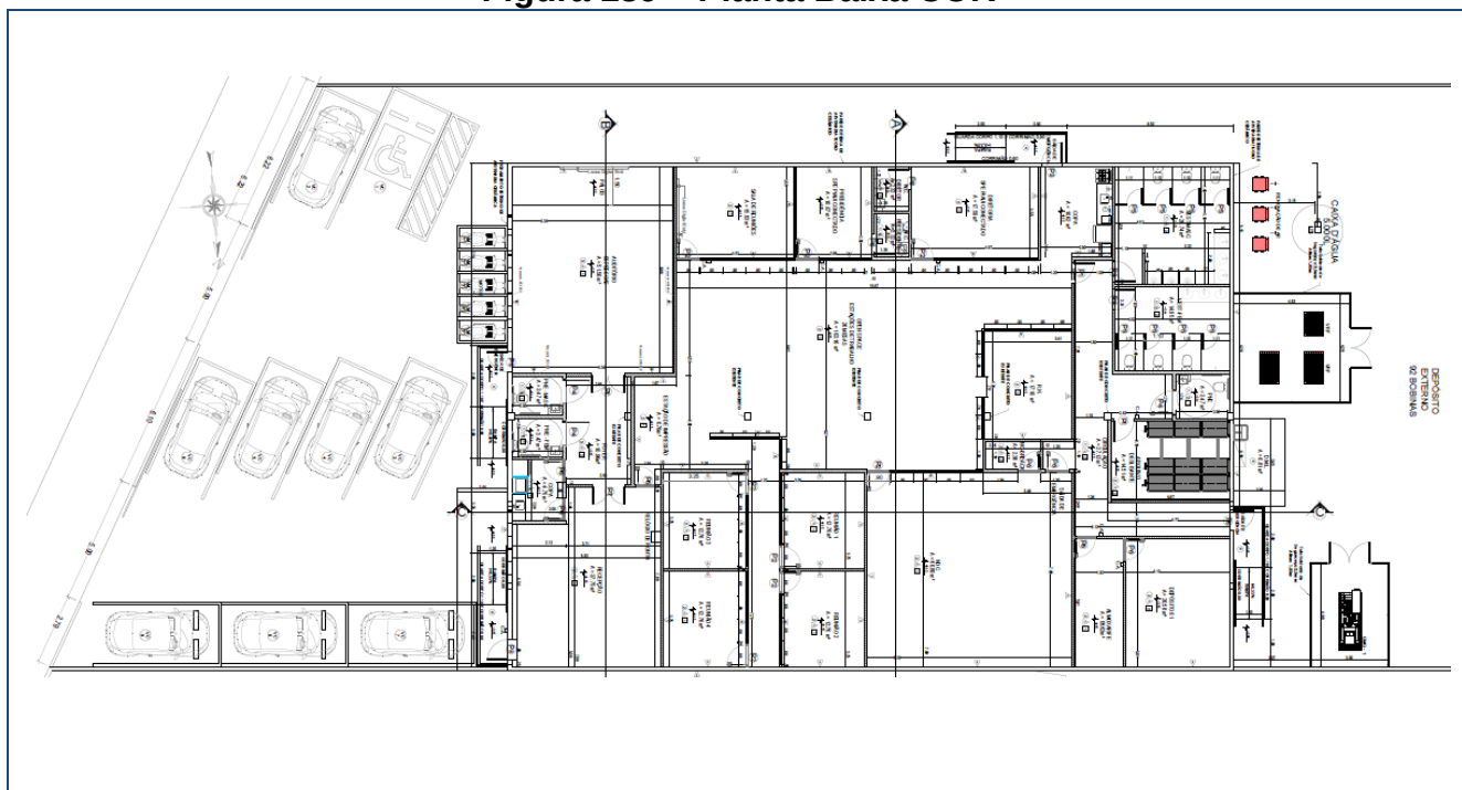
Figura 189 – Planta Baixa COR
