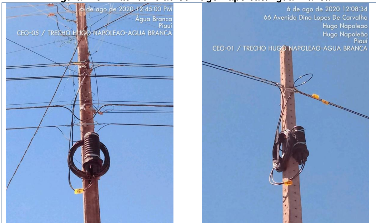
Figura 175 – Backbone aéreo Hugo Napoleão/Água Branca
