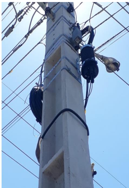
Imagem 4 – CEO já instalada fazendo a junção das fibras nos cabos backbone
